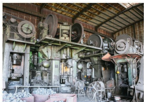
1600吨锻造线 Forging Line
